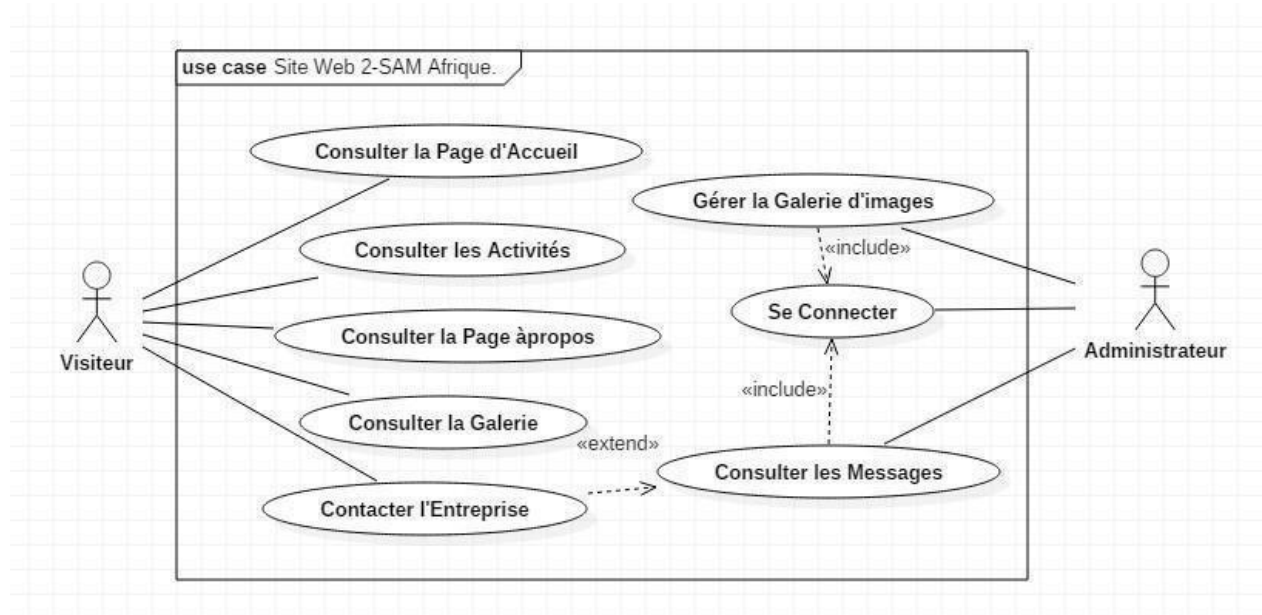
Figure 4: Voici Diagramme De Cas d'Utilisation :
