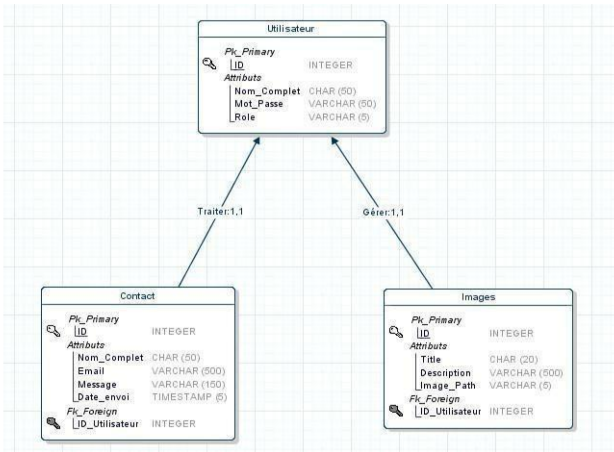
Figure 4 : Voici Le Modèle logique des Données (M.L.D)
