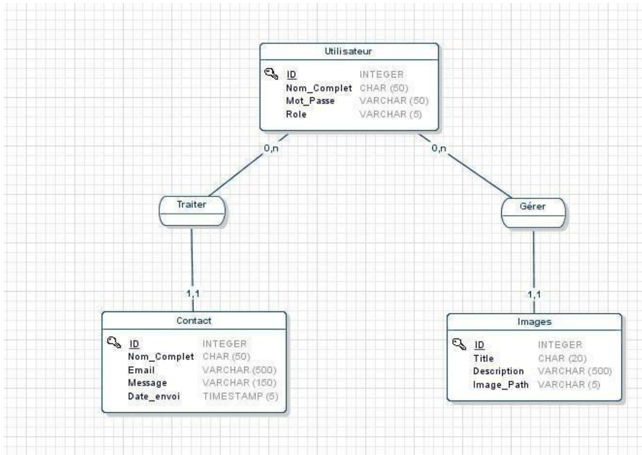
Figure 3 : Voici Le Modèle Conceptuel des Données (M.C.D)
