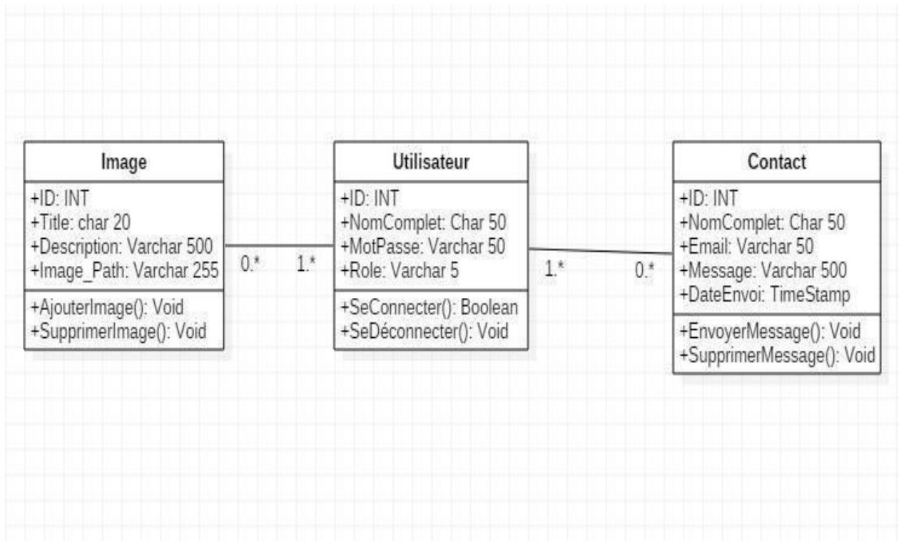
Figure 3 : Voici le Diagramme De Classe
